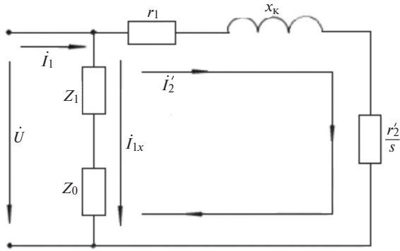
Рис. 1. Г-образная схема замещения одной фазы АД
