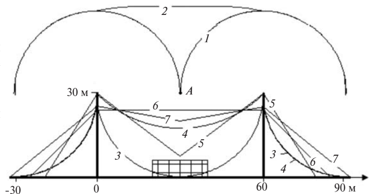
Рис. 2. Зоны захвата (1, 2) и зоны защиты (3–7) двойного молниеотвода с объектом размером 20' 20' 6 м: 1, 3 – МКС; 2, 4 – МНЗ; 5 – ВСП; 6 – СО; 7 – РД (надежность P_H = 0,95 для МКС, МНЗ, ВСП; P_H = 0,99 для СО, зона A для РД)
