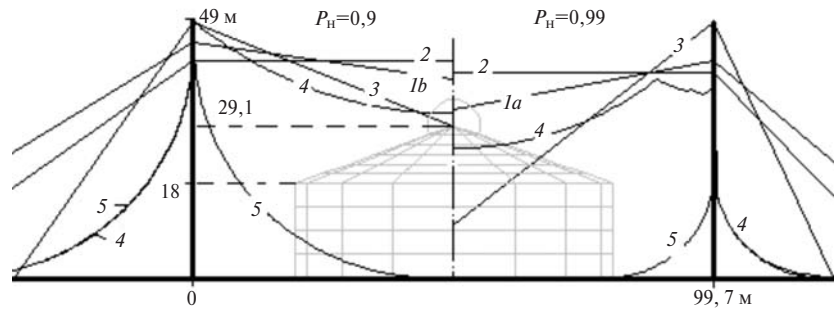
Рис. 4. Зоны защиты резервуара диаметром 60,8 м четырехкратным молниеотводом по: 1а – РД зона А; 1б – РД зона Б; 2 – СО; 3 – ВСП; 4 – МНЗ; 5 – МКС
