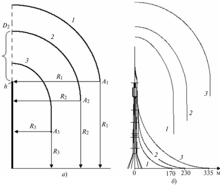
Рис. 3. Зоны захвата молниеотвода (а) при h/D = \text{var} ; зоны захвата и защиты Останкинской башни (б) по МНЗ для тока молнии: 1 – I = 10 \text{ кА} ; 2 – 30 \text{ кА} ; 3 – 100 \text{ кА}
